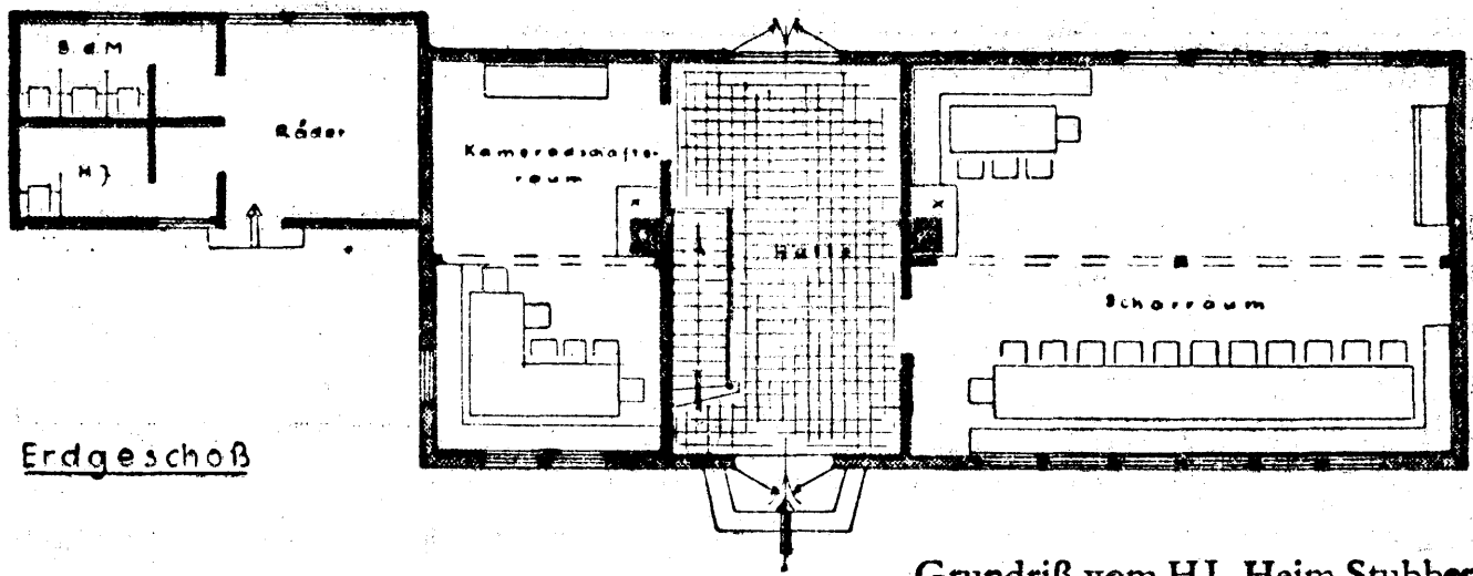
Grundriß vom HJ.-Heim Stubben
