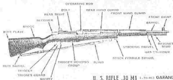
U. S. RIFLE .30 M1 (1-39-00) GARAND
