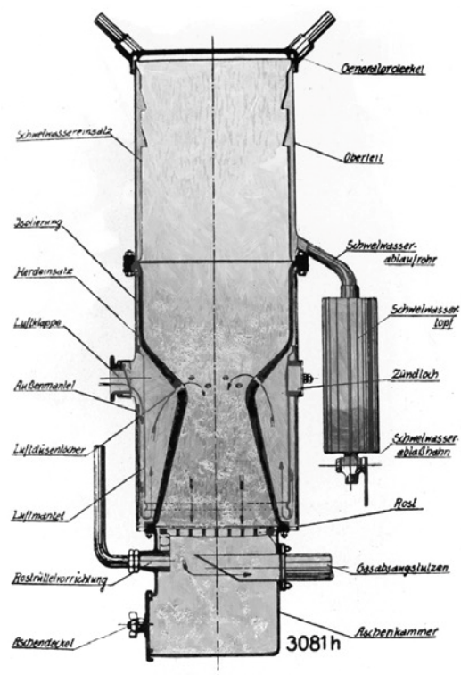
Bild 8. Kromag-Holzgasleingenerator Type „K“
