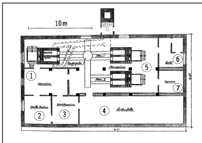
Obr. 1: Půdorys krematoria I v hlavním táboře Osvětím I v původním stavu. Márnice se později údajně měla používat jako „plynová komora“.
