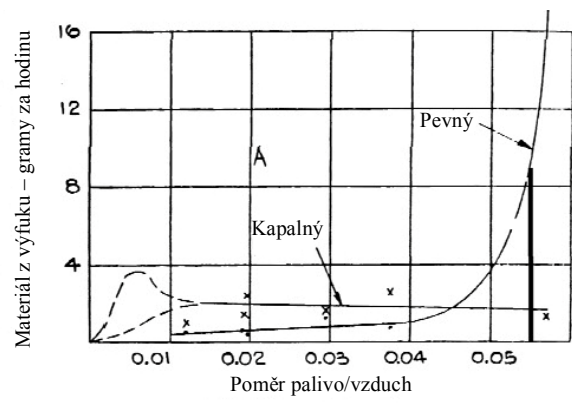
Graf 7: Kapalně a pevně látky ve zplodinách z motoru za hodinu a množství kouře. 1894 Silná svislá čára označující poměr palivo/vzduch 0,055 (vzduch/palivo 18 : 1) doplněna autorem.
