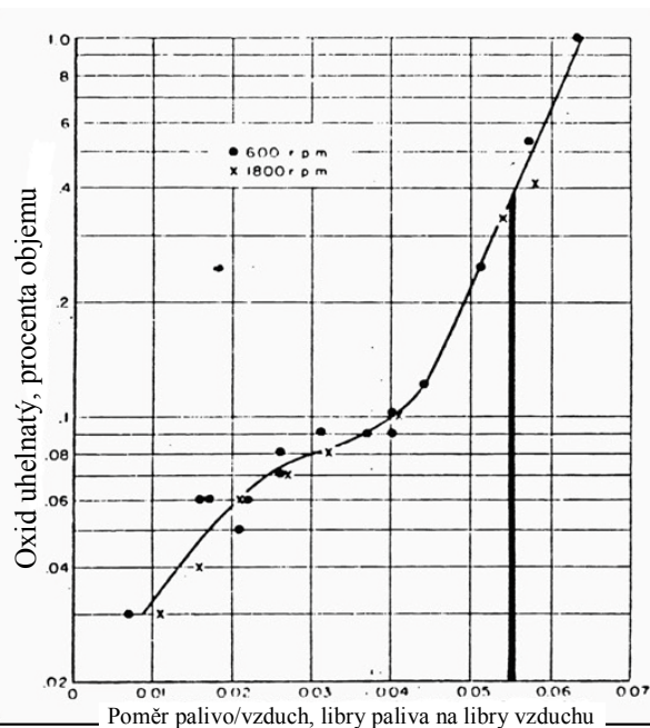
Graf 5 (nahore): Emise CO z dieselu s neděleným spalovacím prostorem (C). 1870
