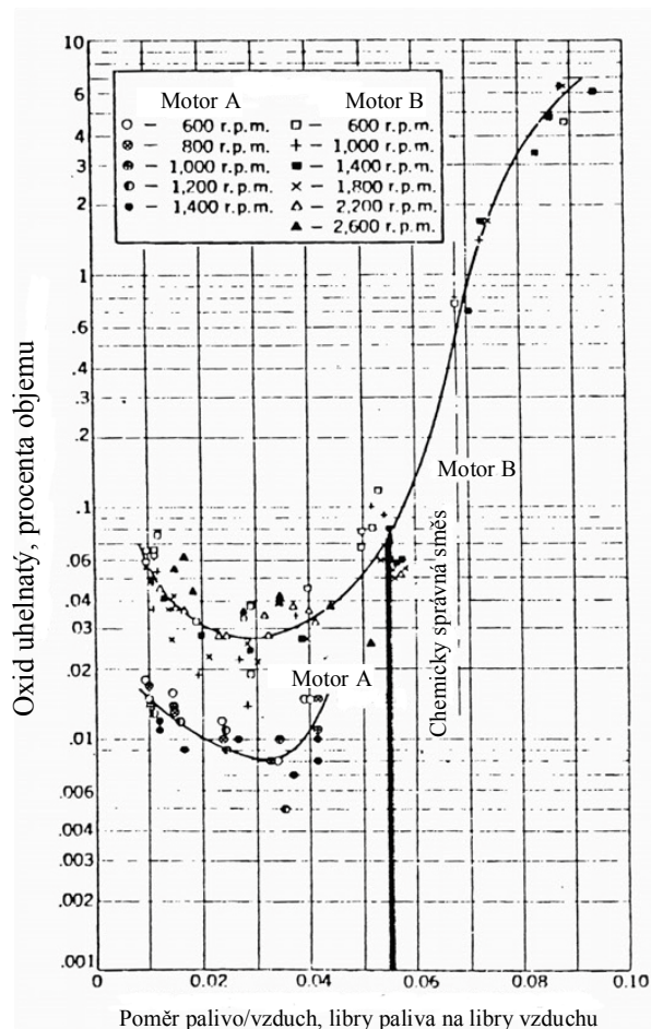
Graf 5 (nahore): Emise CO z dieselu s neděleným spalovacím prostorem (C). 1870
