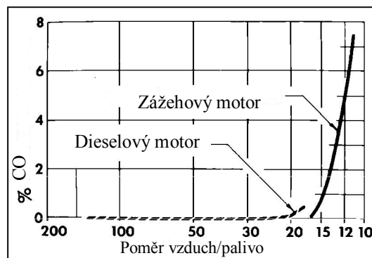
Graf 3: Emise CO z diesellových a spalovacích motorů. 1869
