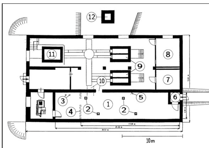
Obr. 2: Půdorys krematoria I v Osvětím I (hlavním táboře) dnes, po poválečných úpravách.
