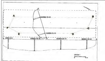
Ryc. 18. Dół śmierci nr 1. Plan oraz przekroje grobu (na podstawie archeologicznych sondażów wiertniczych)
