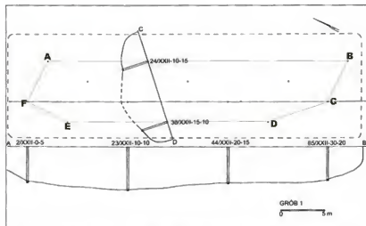
Ryc. 18. Dół śmierci nr 1. Plan oraz przekroje grobu (na podstawie archeologicznych sondażi wiertniczych)
